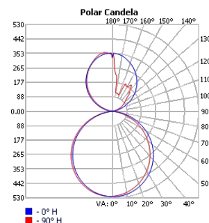
TECHOLED-BX-2-DI-2-HI-30
